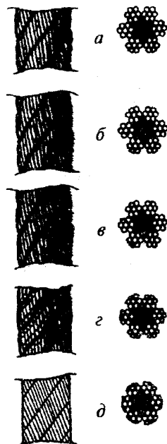
Рис. 5. Износ наружных проволок каната крестовой свивки: a — небольшие лыски на проволоках; б — увеличенная длина лысок на отдельных проволоках; в — удлинение лысок в отдельных проволоках при заметном уменьшении диаметра проволок; г — лыски на всех проволоках, уменьшение диаметра каната; д — интенсивный износ всех наружных проволок каната (уменьшение диаметра проволок на 40%)
